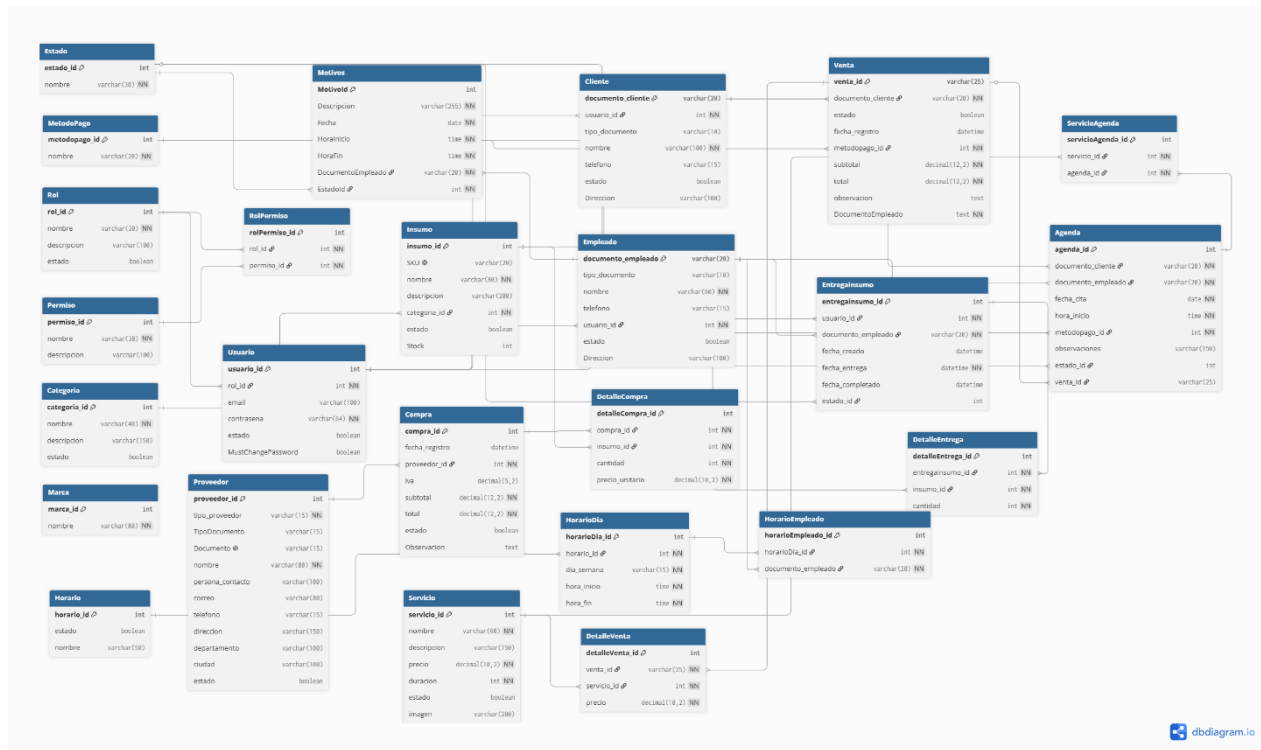
Figura 40. Modelo relacional
