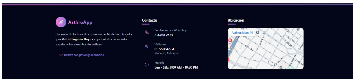
Figura 39. Prototipo Footer
