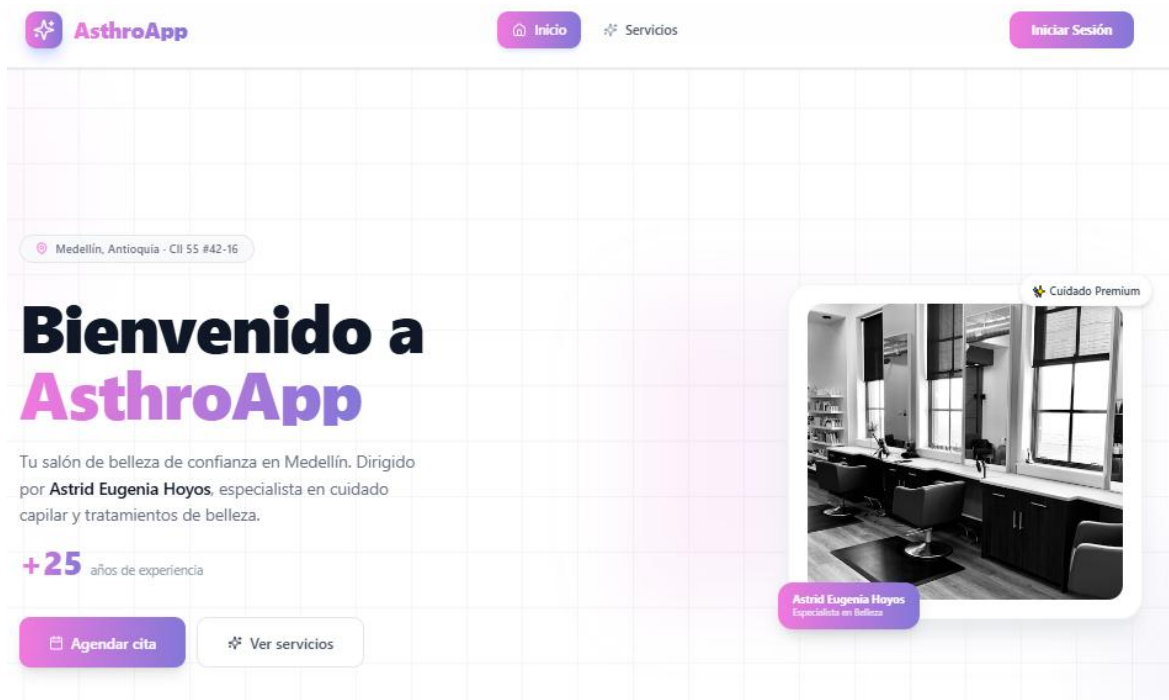
Figura 37. Prototipo Landing
